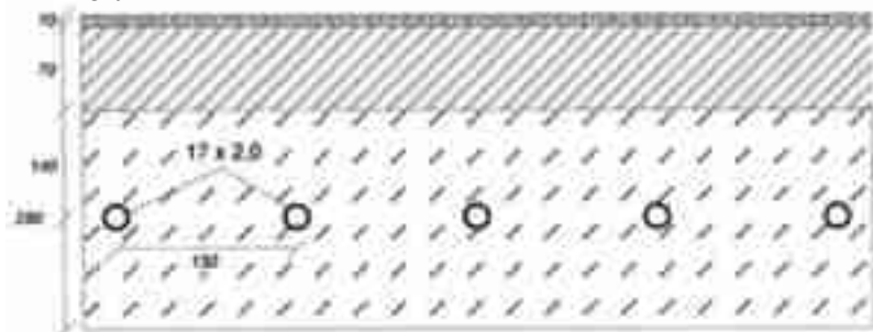
Slika 5 Vgradnja cevi za temperiranje betonskega jedra
