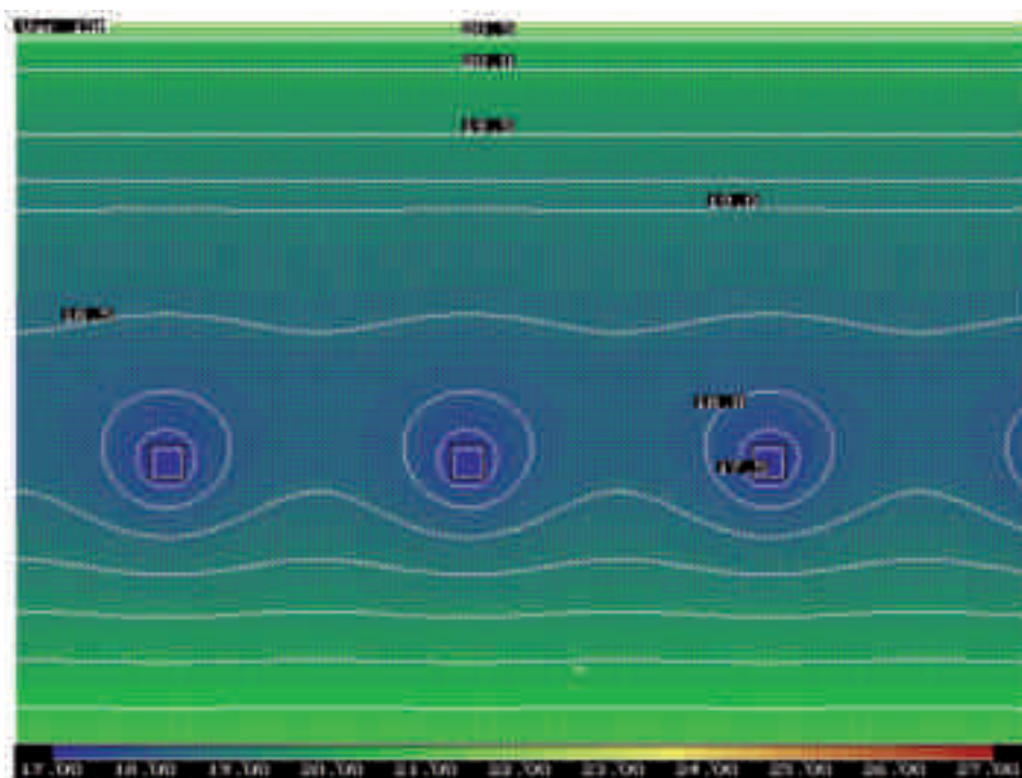
Slika 6 Temperature pri hlajenju s temperiranjem betonskega jedra
