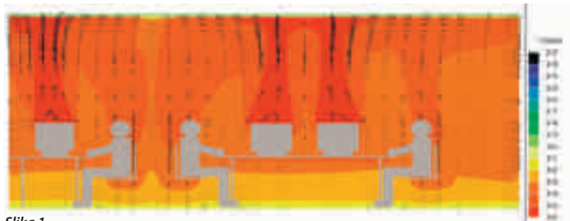
Slika 1 Temperaturne razmere pri temperiranju betonskega jedra in prezračevanju skozi okna
